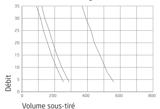
Courbes de sous tirage Entrée eau 15°C
